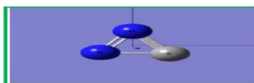
ChemNewsNew (CNN)
